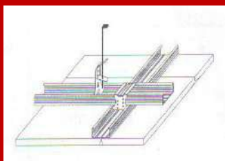
Strop spuščeni D112 m2
