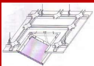
Revizijska loputa montaža D171 kos
