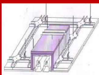
Obloga svetil z pož.ploščo D181 m1
