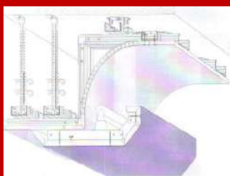
Stropna nadsvetlobna polica do 20cm m1
